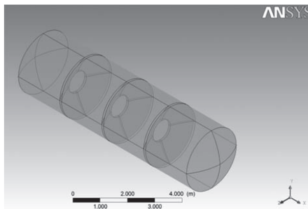
Рисунок 7 — Модель резервуара цистерны с перегородками сферической формы
