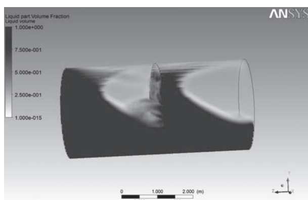
Рисунок 6 — Перетекание жидкости через перфорированную перегородку
