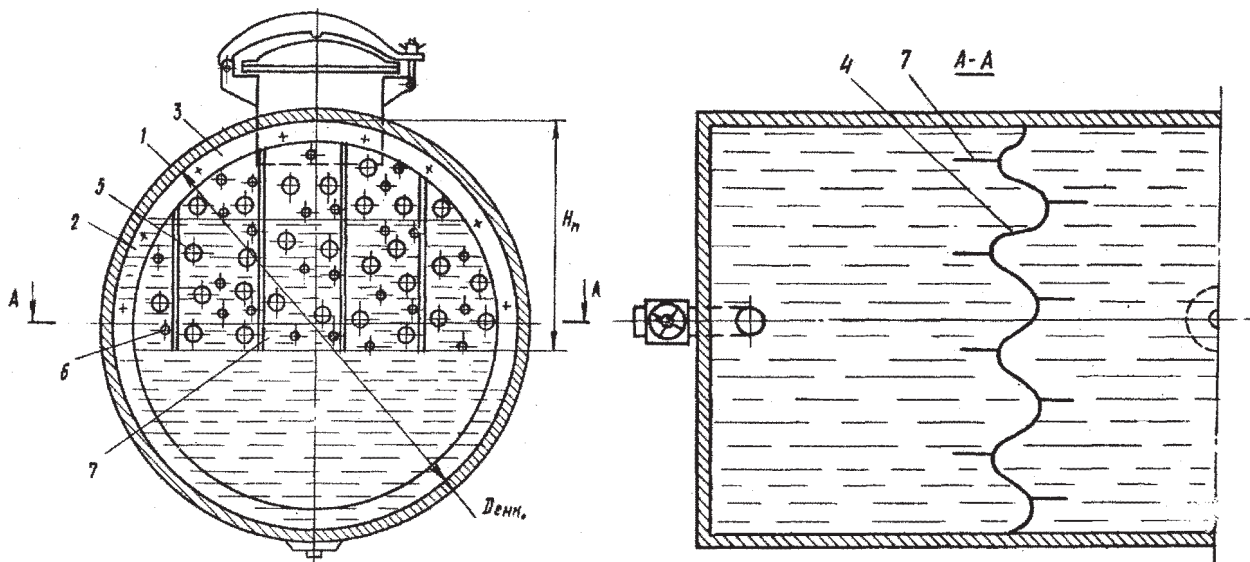
Рисунок 1 — Цистерна с гофрированными волнорезами SU 0981121 [3]
