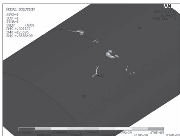
Рисунок 10 — Схема распределения напряжений в резервуаре с перегородкой, изготавливаемой на ГМЗ в настоящее время
