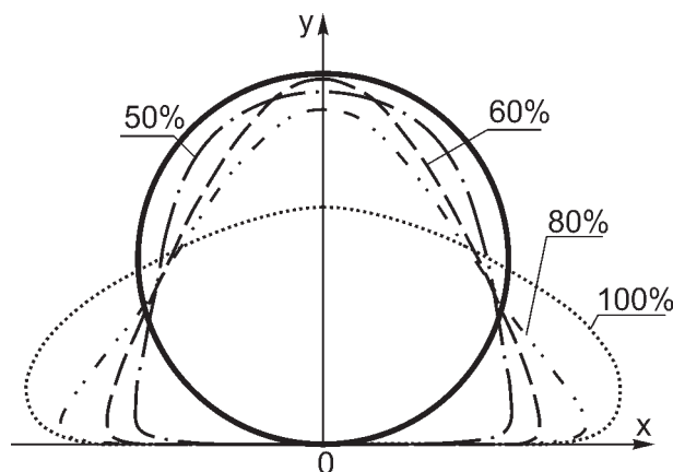
Рисунок 4 — Результаты оптимизации формы резервуара цистерны при различных уровнях заполнения
