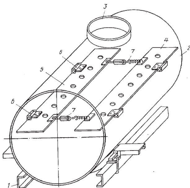
Рисунок 3 — Цистерна с шарнирно закрепленными горизонтальными перегородками по изобретению SU 1270056 [7]
