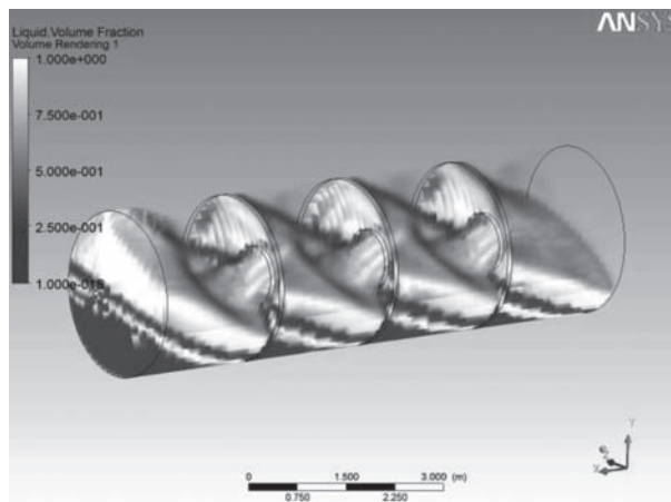
Рисунок 8 — Перетекание жидкости через отверстия в перегородках при одновременном повороте и торможении в момент 0,75 с после начала движения цистерны
