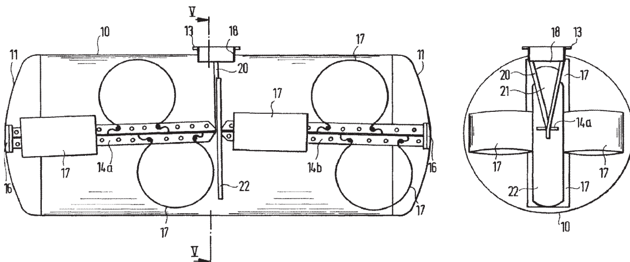
Рисунок 2 — Цистерна с \Omega -образными обечайками по патенту EP 212653 [4]
