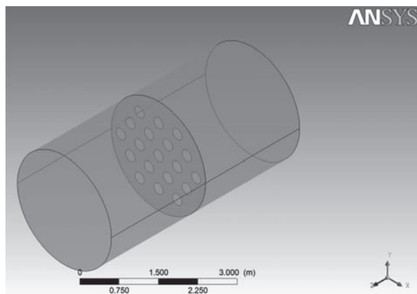
Рисунок 5 — Модель резервуара цистерны с перфорированной перегородкой
